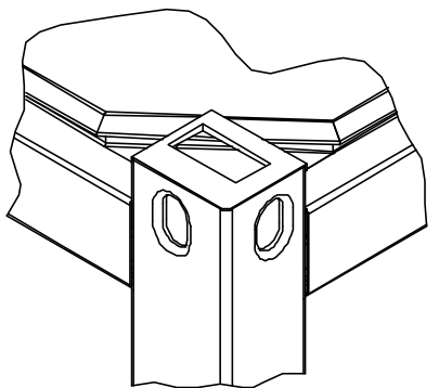
Ansicht P: (M 1:5)
